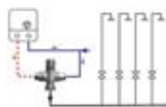
TMTCOM Termostatický směšovač 1" 4 až 8 odběrných míst, 20-50 °C, F1"xF3/4" zpětná klapka, filtr 3 490,- / 145 €
